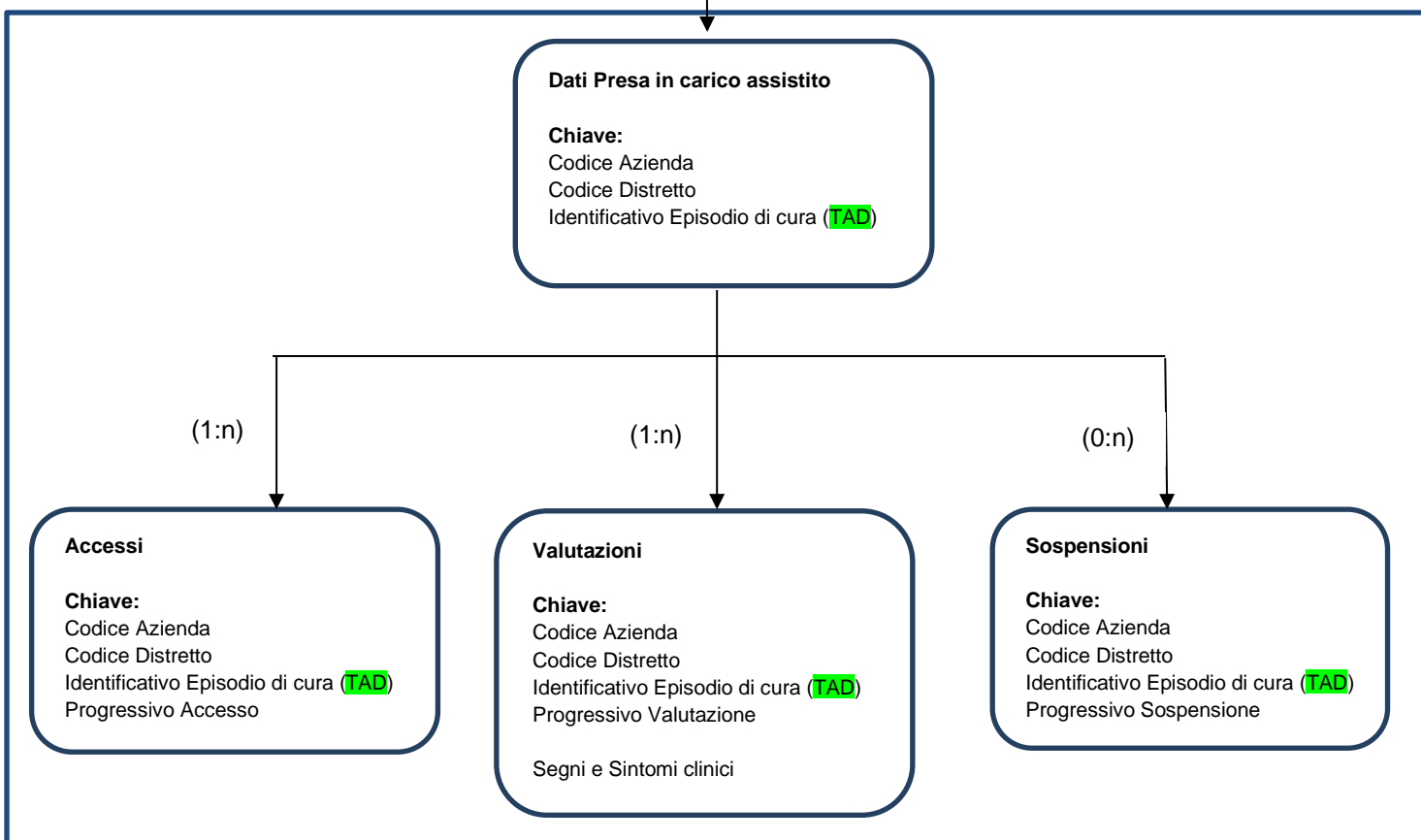
Figura 1 - Schema relazionale
